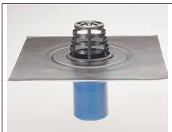
Receptor de garaj/balcon DN 70 cu guler adeziv și ieșire verticală
